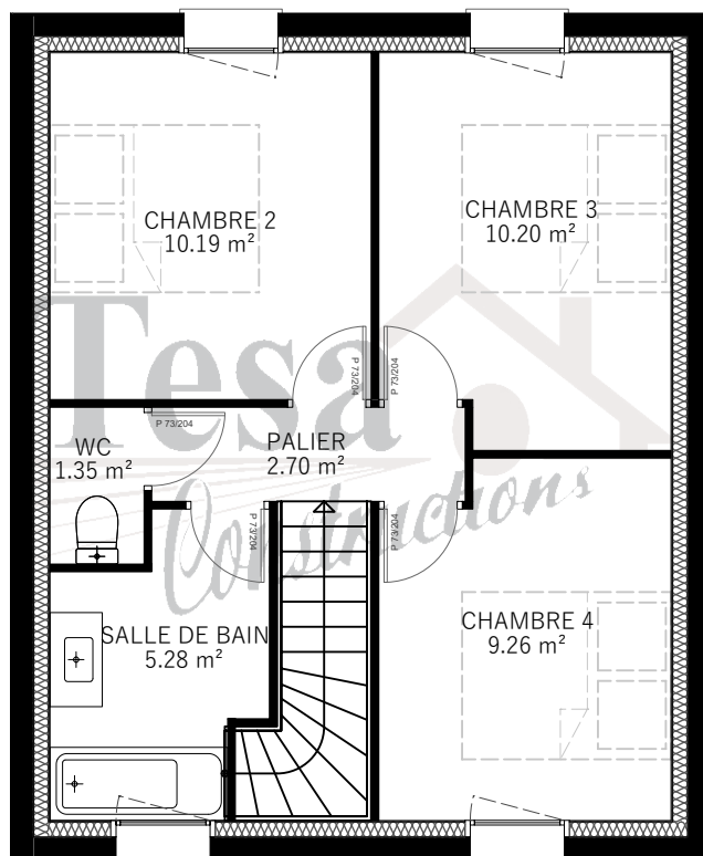
ÉTAGE
